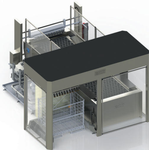
Bac de congélation linéaire BGL 2000
