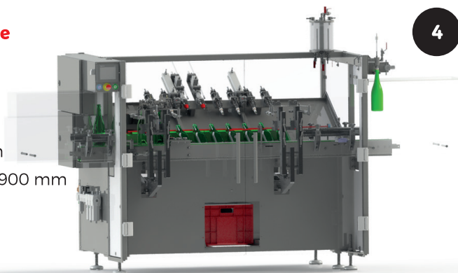
Boucheuse - Museleuse automatique FRANVAL 1000
